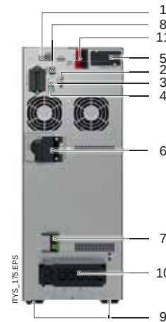
ITYS 6 - 10 kVA - 1/1
