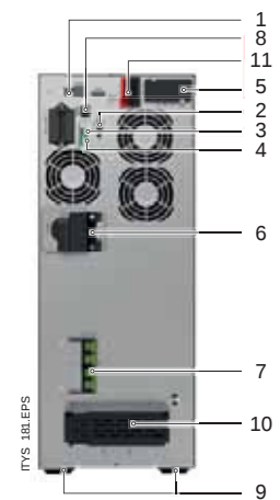
ITYS 8.5 - 10 kVA - 1/1 or 3/1
