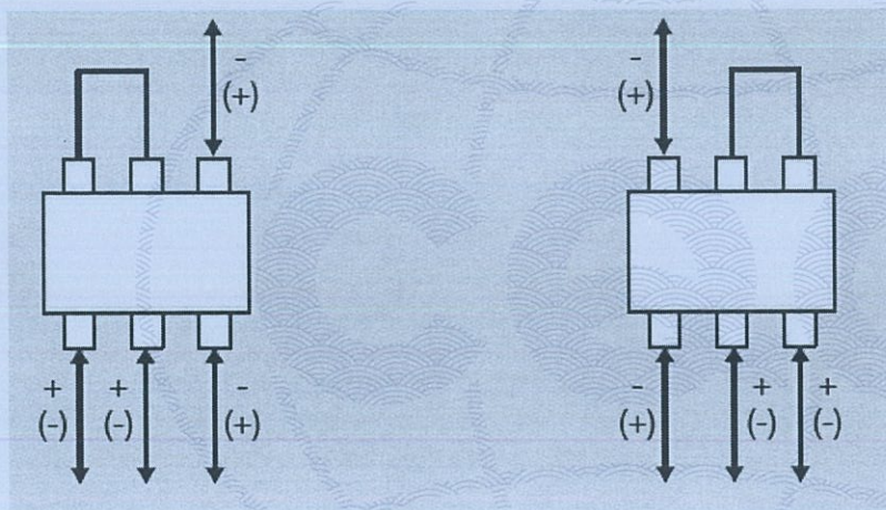
直流接线图
