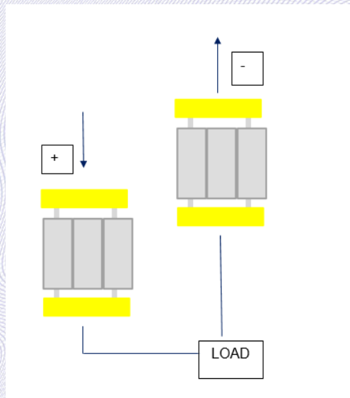
接线方式1
