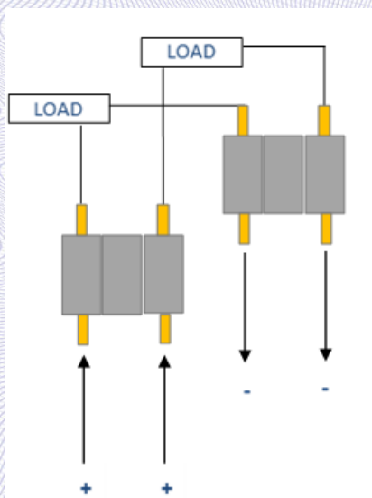
接线方式2
