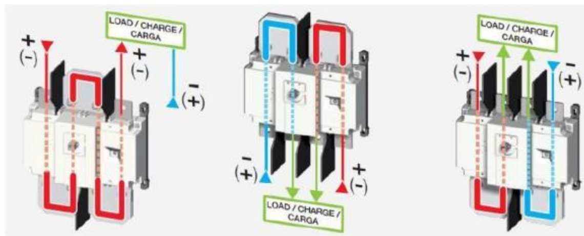
接线方式 1
