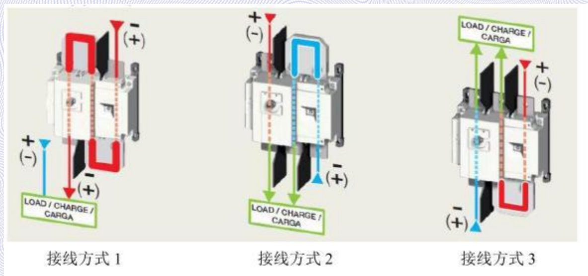
750V DC 3P 外形接线图
