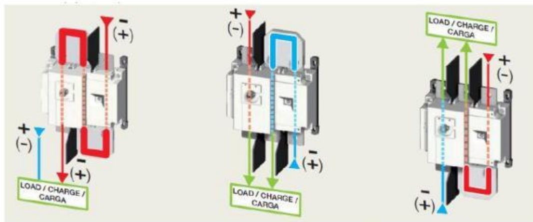
接线方式1
