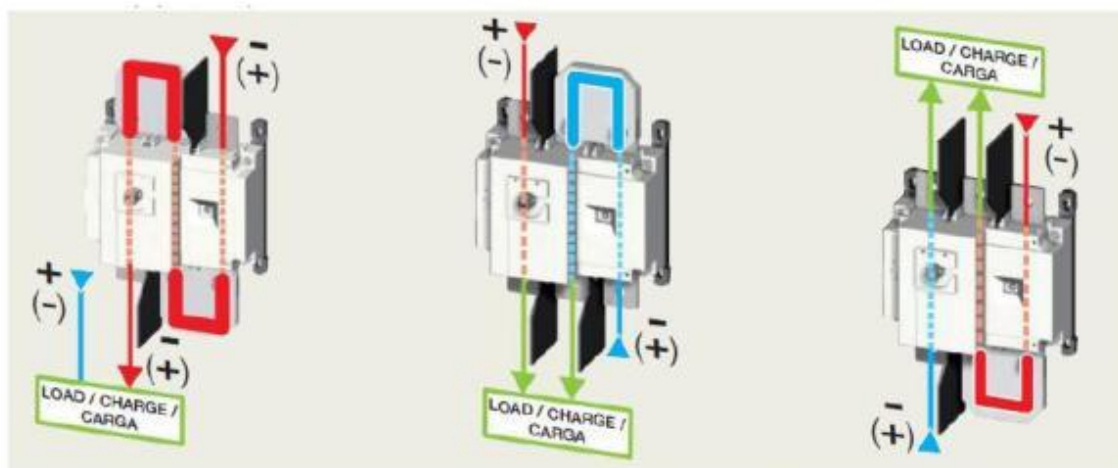
接线方式1
