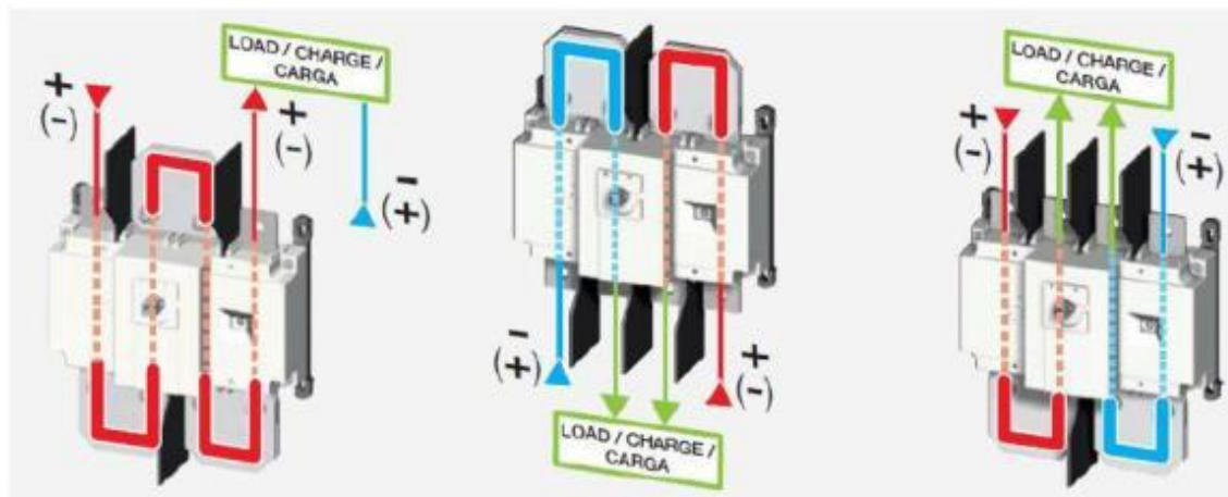
接线方式1
